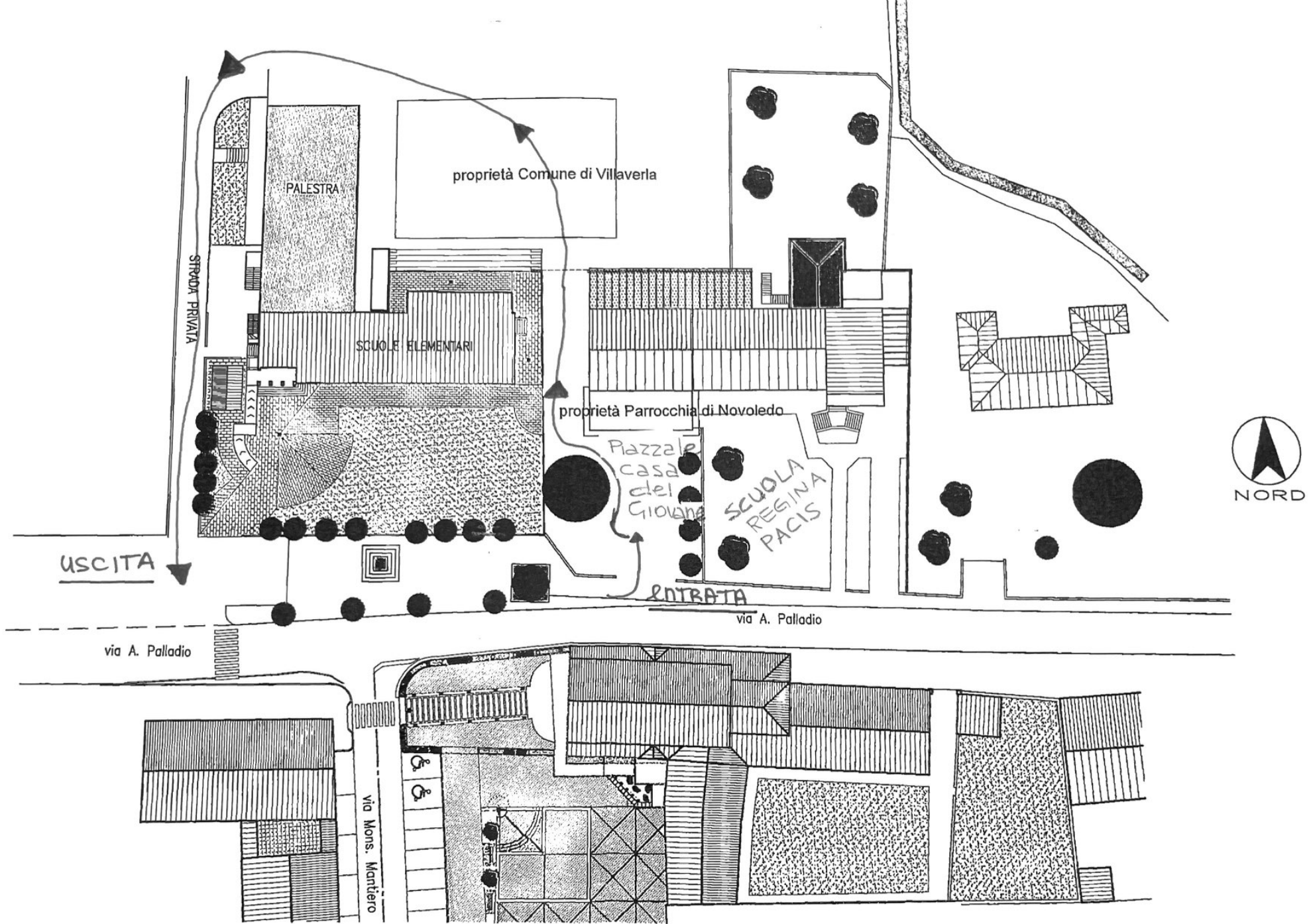
PLANIMETRIA - scala 1:500
